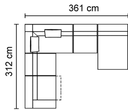
175 SECT.(450+01+32+01+49)
